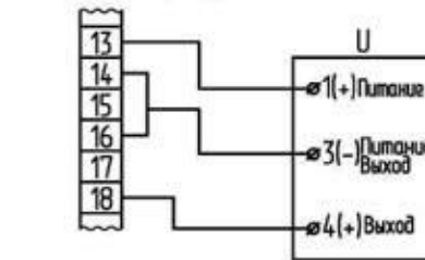
Рисунок Б.5-Схема механизма МЭО-92К с БСПТ-10М; Остальное - см. рисунок Б.2
