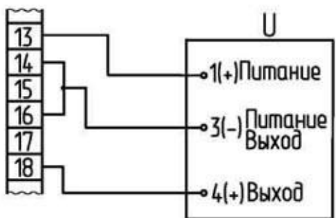
Рисунок В.5 - Схема с БСПТ-10М Остальное - см. рисунки В.1 или В.2
