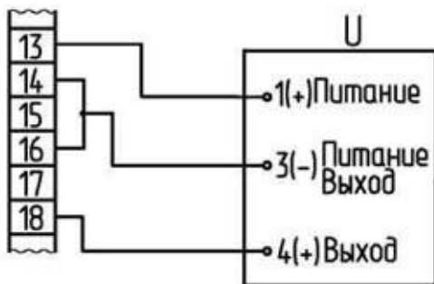
Рисунок В.5 - Схема с БСПТ-10М Остальное - см. рисунки В.1 или В.2
