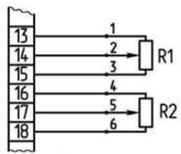
Рисунок В.4 - Схема с БСПР-10 Остальное - см. рисунки В.1 или В.2
