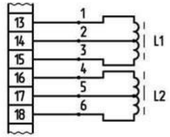
Рисунок В.3 - Схема с БСПИ-10 Остальное - см. рисунки В.1 или В.2
